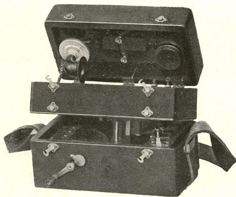
Types d'appareils pour installations à appel magnétique.
