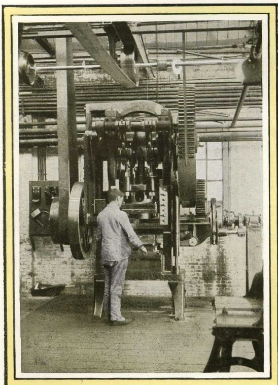
Travail d'estampage.
