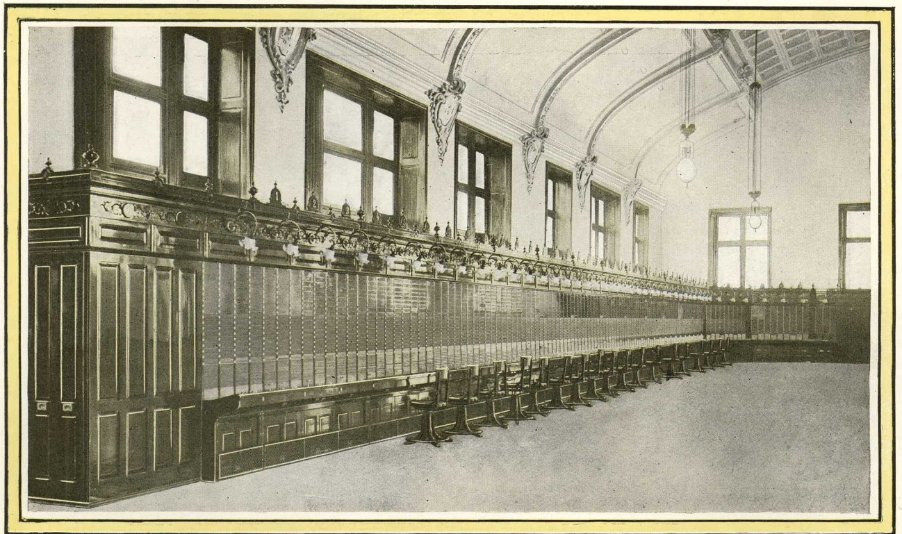
Installation caractéristique à batterie centrale. Bureau central d'Anvers.
