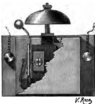
FIG. 35. — Sonnerie trembleuse.
