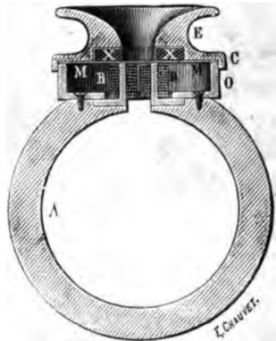
FIG. 11. — Coupe du récepteur Ader.
