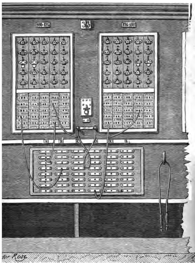
FIG. 26. — Commutateur.
