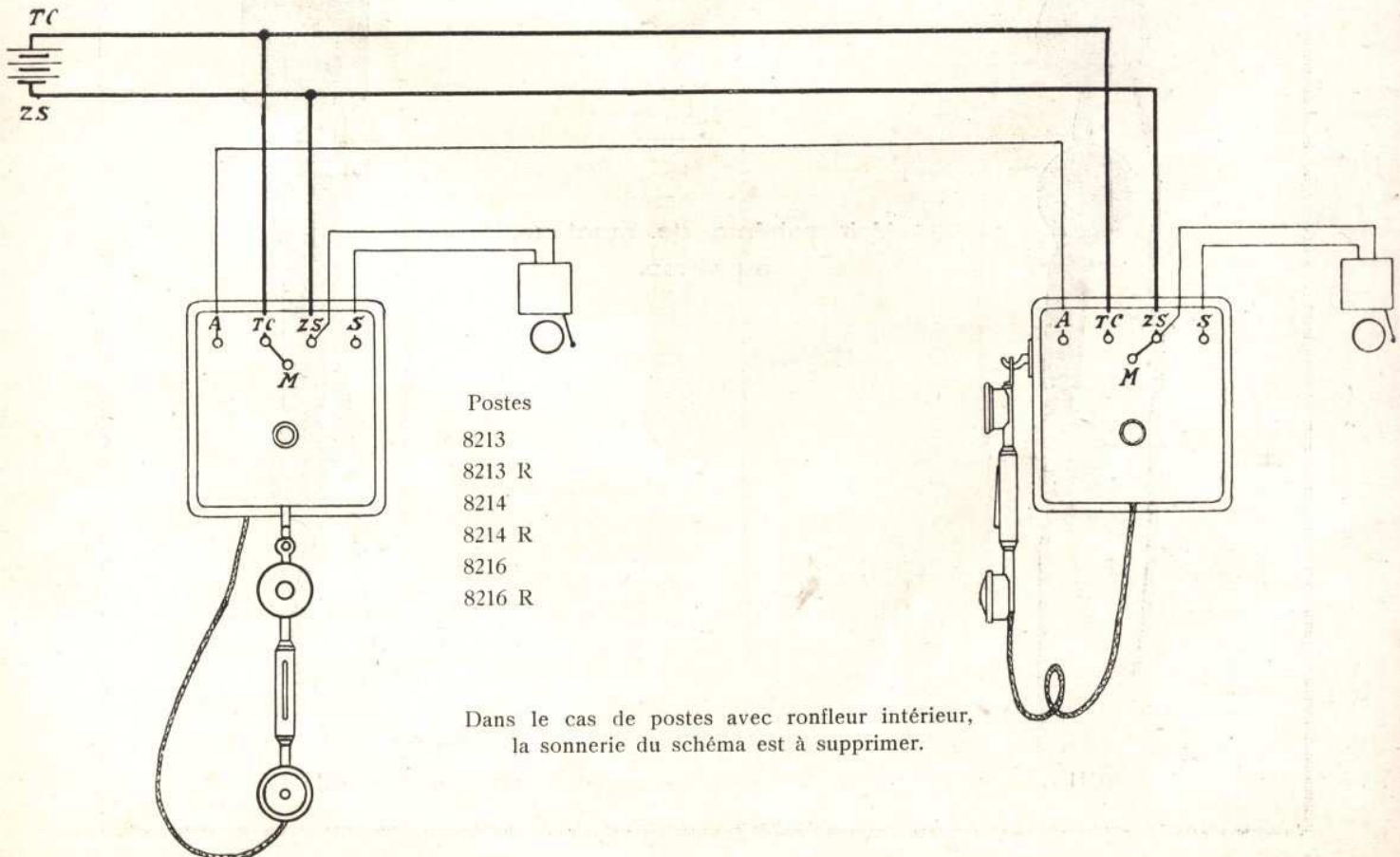
Schéma d'installation de 2 postes à appel réciproque
