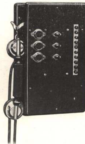
Poste mixte mural, à 3 lignes réseau B. C. I., 10 lignes privées
