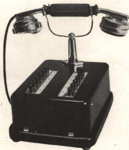
Poste mobile à 12 directions 2200 P. 12
