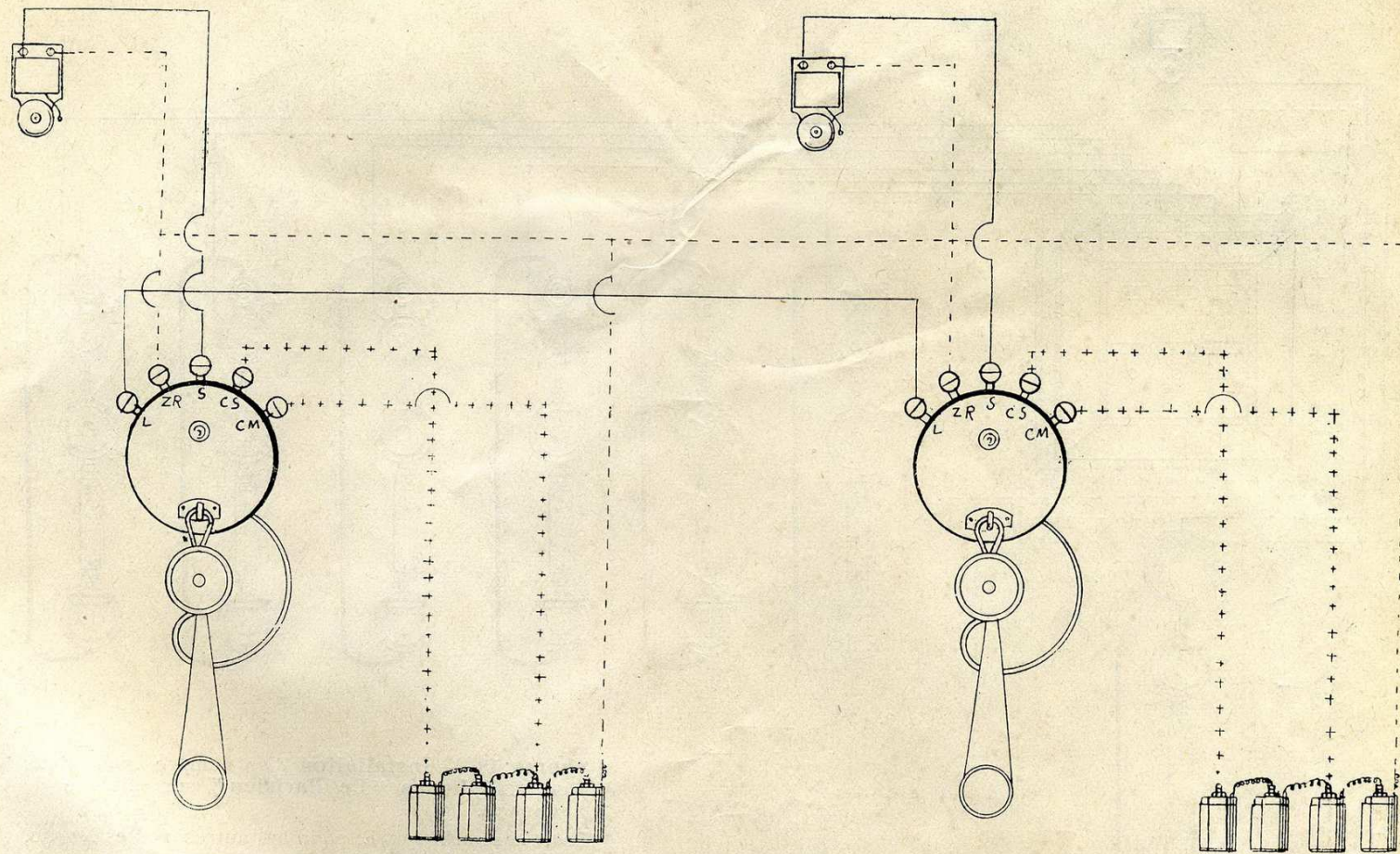
Schéma 28. — Installation de 2 postes le "Soliphone" à circuit secondaire N os 608 et 609.
