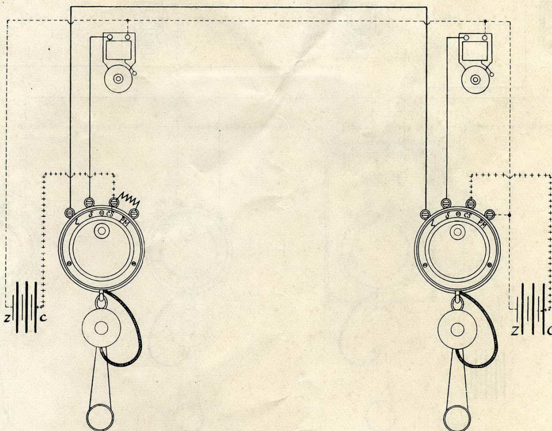
Schéma n° 5. — Installation de 2 postes par 2 fils et 2 batteries, postes primaires à crochet commutateur nos 541-542 et "Parisien" 532-I.
