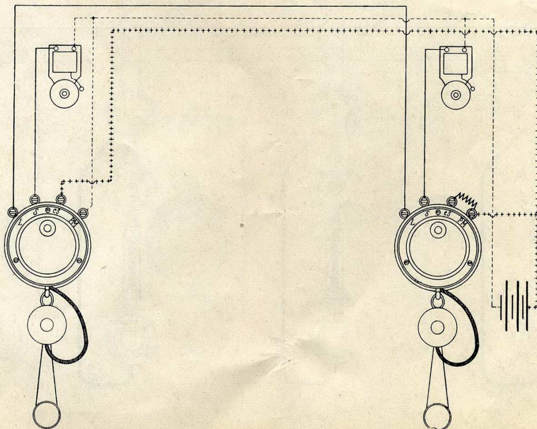
Schéma n° 6. — Installation de 2 postes par 3 fils et 1 batterie, pour postes primaires à crochet commutateur nos 541-542 et "Parisien" 532-I.
