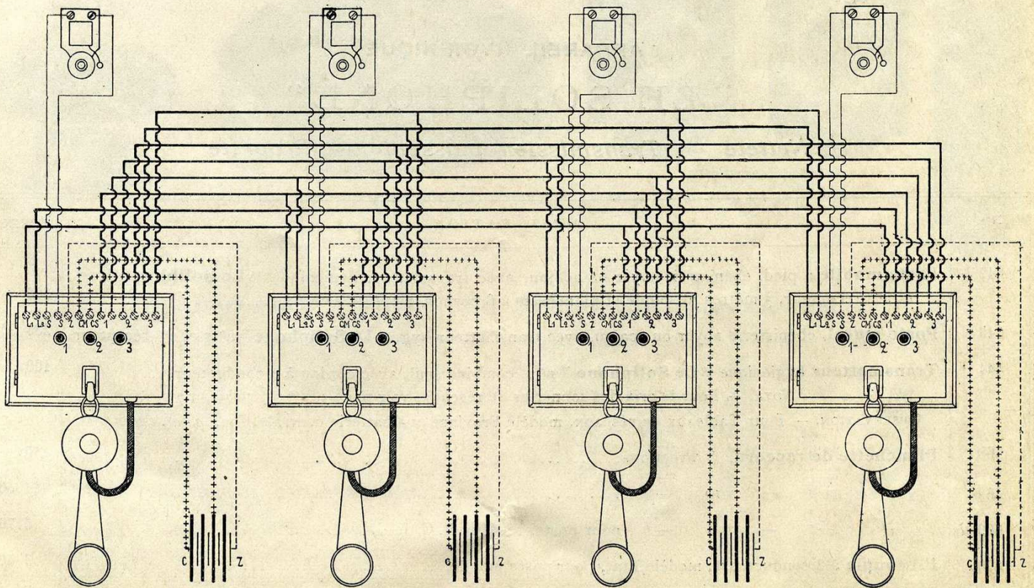
Schéma n° 54. — Installation d'un nombre quelconque de postes "REMISE AUTOMATIQUE A ZÉRO" à circuit secondaire (montage au double fil), à intercommunication), permettant la conversation simultanée de plusieurs paires de postes entre eux. La conversation des uns n'est pas troublée par celle des autres.
