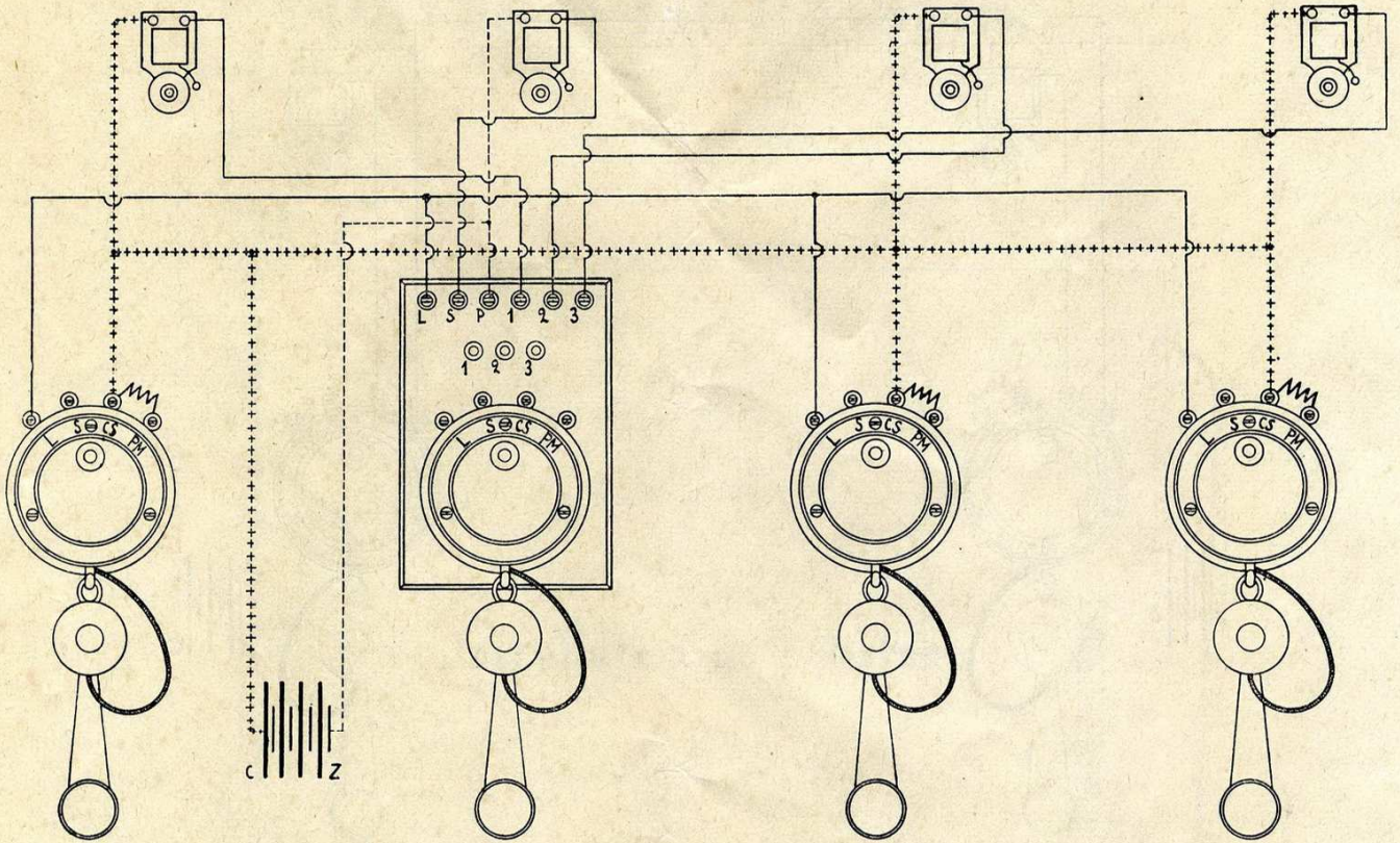
Schéma n° 11. — Installation de postes nos 541-542 et " Parisiens " 532-I dont un forme central.
