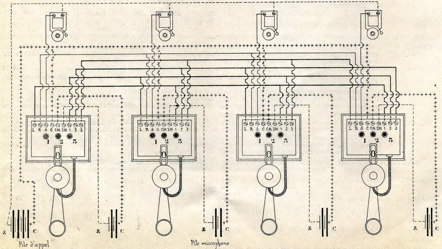
Schéma N° 52. — Installation d'un nombre quelconque de postes "REMISE AUTOMATIQUE A ZÉRO", à circuit primaire, à intercommunication permettant la conversation simultanée de plusieurs paires de postes entre eux. La conversation des uns n'est pas troublée par celle des autres.
