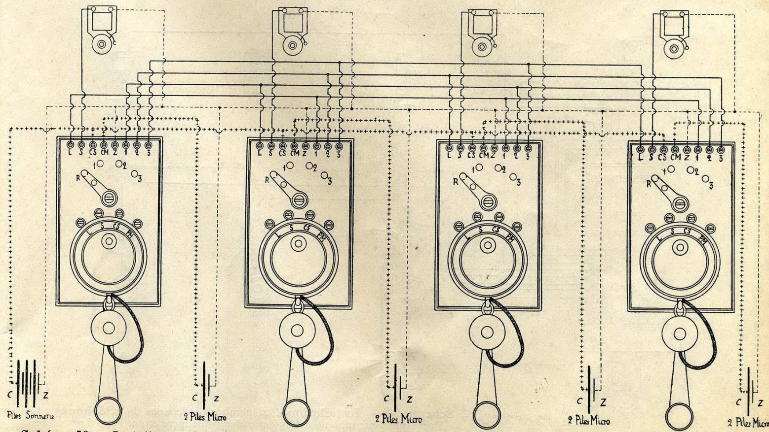
Schéma 50. — Installation de postes "Soliphones" n os 541 et 542, communiquant entre eux, avec combinateurs n os 586 S et 587 S bis. Une batterie d'appel et une pile micro par poste, permettant de pouvoir faire converser plusieurs paires de postes en même temps.
