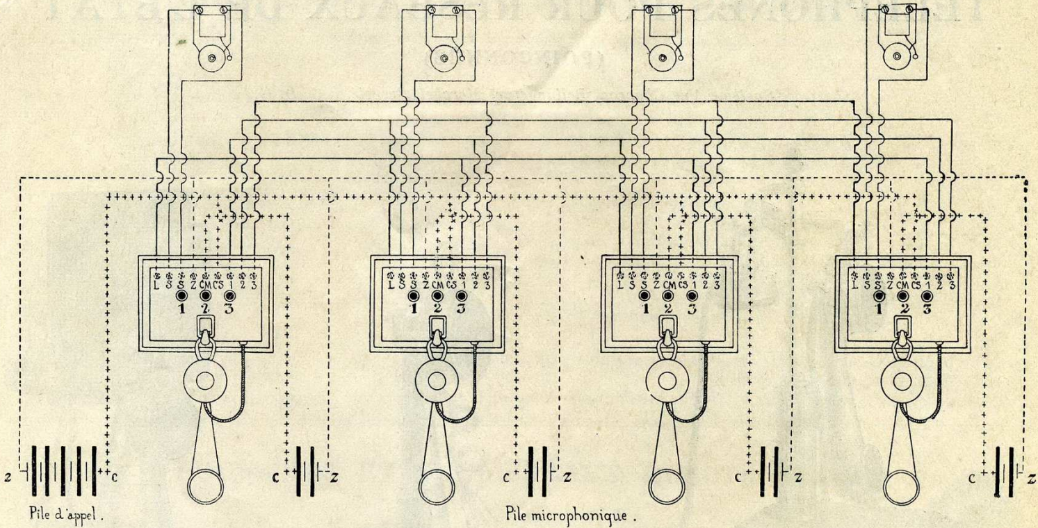
Schéma n° 53. — Installation d'un nombre quelconque de postes "REMISE AUTOMATIQUE A ZÉRO" à circuit secondaire (montage au simple fil), à intercommunication), permettant la conversation simultanée de plusieurs paires de postes entre eux.
