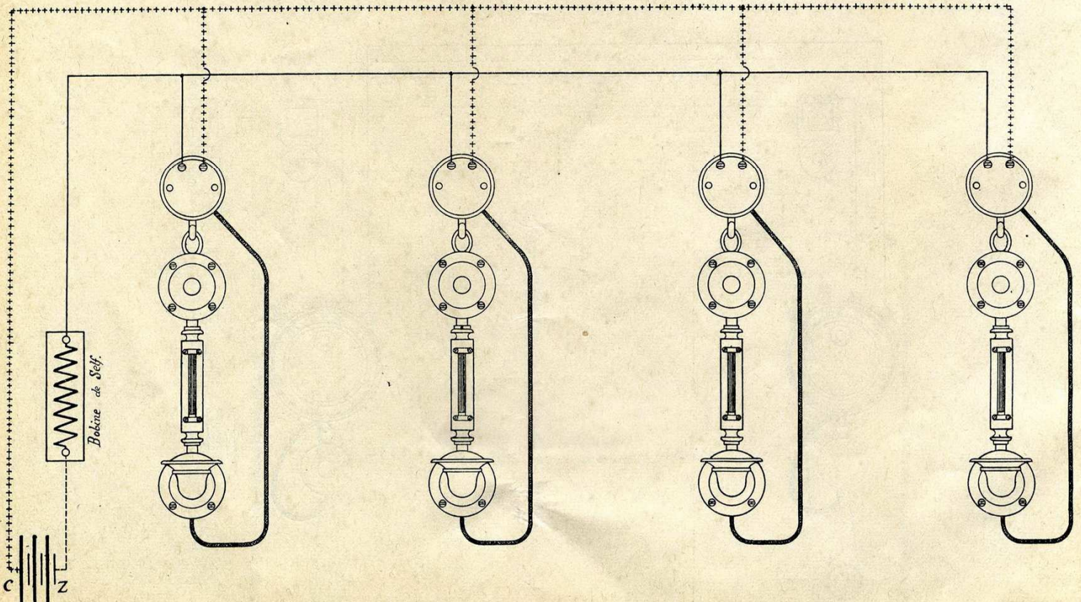
Schéma n° 55. — Installation d'un nombre quelconque de postes " Le Parisien " 530 A, embrochés avec bobine de self et appels de sonnerie indépendants.
