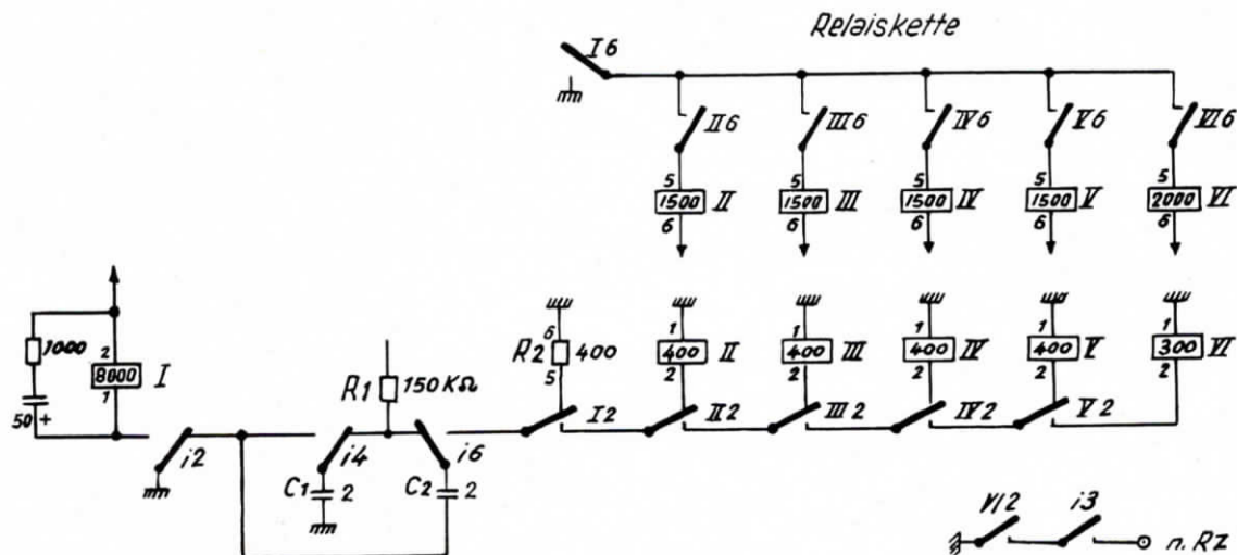
Abb. 3 Die Relaiskette
