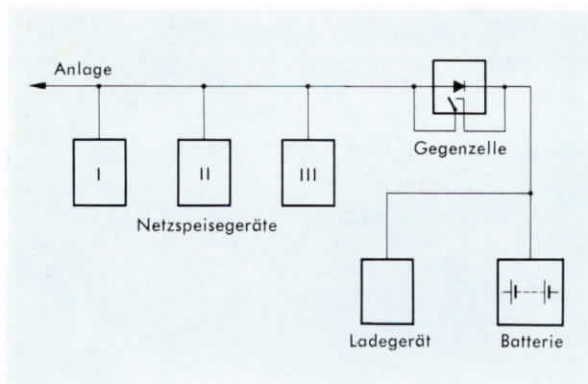
BILD 5 Prinzipschaltbild der Netzspeisung
