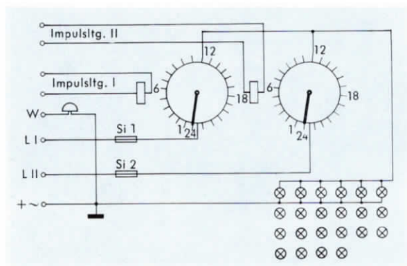
BILD 6 Prinzipschaltbild der Personensucheinrichtung
