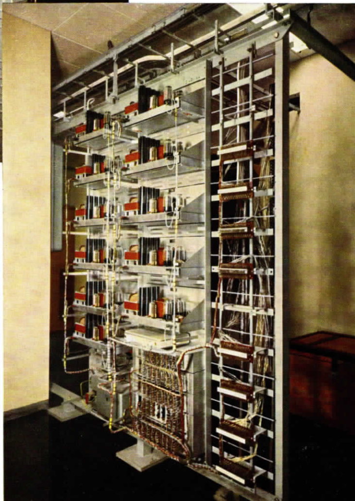
BILD 15 Elektro-akustische Verstärkerzentrale
