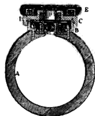
FIG. 2. — Récepteur Ader n° 1. Coupe transversale.
