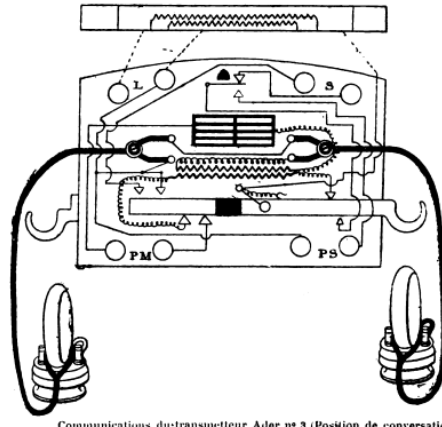
Communications du transmetteur Ader n° 3 (Position de conversation).
