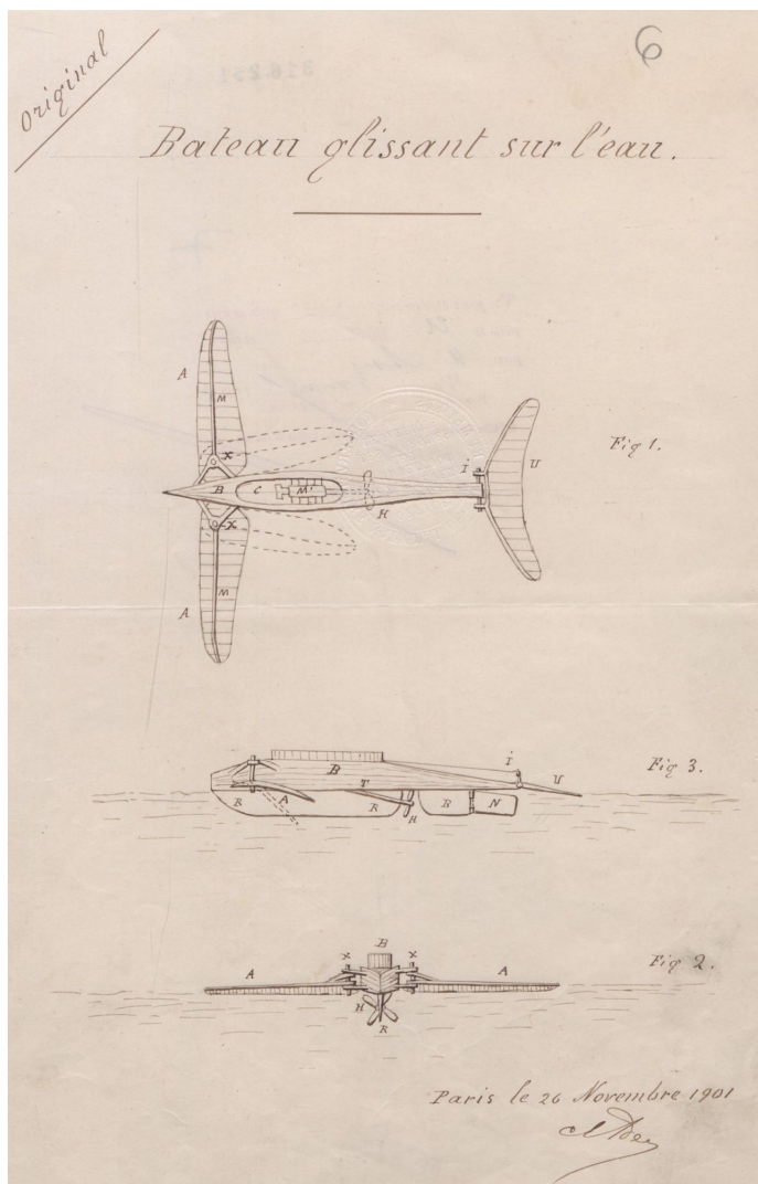
Brevet n°316251 déposé le 26.11.1901 pour un "bateau glissant sur l'eau".
