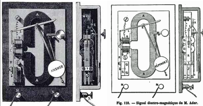
Fig. 118. — Signal électro-magnétique de M. Ader.
