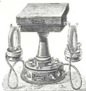
FIG. 38. — Transmetteur Ader, type n° 4.
