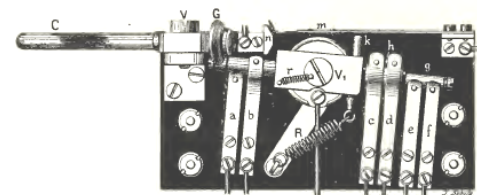
Fig. 35. — Levier-commutateur du transmetteur Ader.
