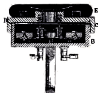
FIG. 4. — Récepteur Ader n° 3. Coupe transversale.
