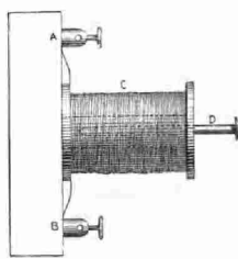
Fig. 102. — Téléphone sans noyau de fer de M. Ader.
