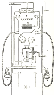
FIG. 104. — Schéma des connexions de l'appareil avec appel magnétique de la Société Industrielle des Téléphones.
