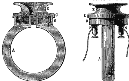
Fig. 2 - Téléphone Ader. (Coupe longitudinale.) Fig. 3 - Téléphone Ader. (Vue de Côté) fabriqué en premier par Ladislas Lenczewski et Cie
