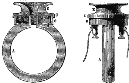
Fig. 2 - Téléphone Ader. (Coupe longitudinale.) Fig. 3 - Téléphone Ader. (Vue de Côté)
