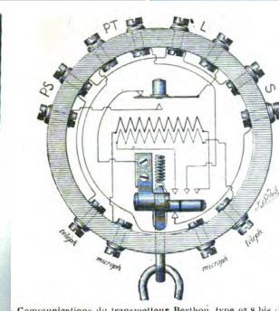
Communications du transmetteur Berthon, type n° 8 bis (Position d'appel).
