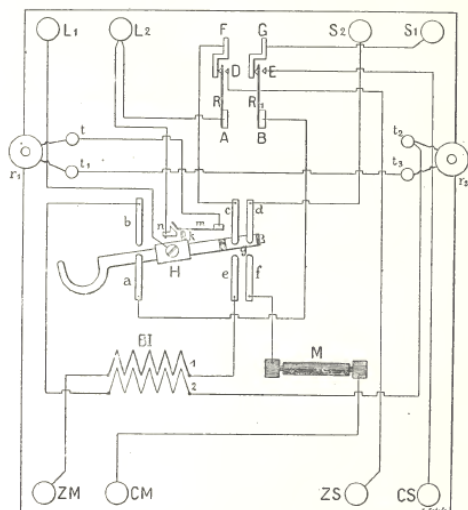
FIG. 36. — Schéma des connexions du transmetteur Ader.
