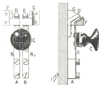
FIG. 34. — Clé d'appel du transmetteur Ader.
