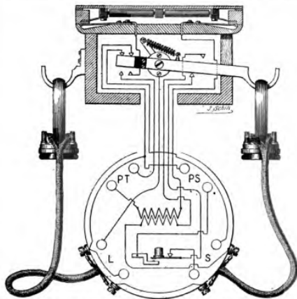
Fig. 34. — Communications du transmetteur Ader n° 4 (Position d'appel).
