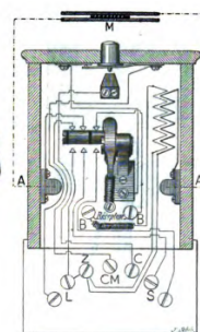
Fig. 196. — Communications du transmetteur Berthon, forme cartel (Position de conversation).
