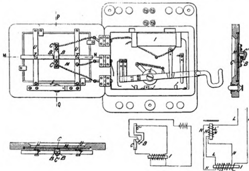
Fig. 1 à 5. — Microphone Ader. Élévation, coupes M N, P Q, et schémas des connexions.
