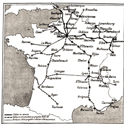
1920 — Réseau des câbles téléphoniques souterrains français.
