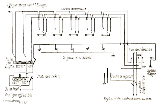
Fig. 1. — Ligne d'appel des annotatrices.
