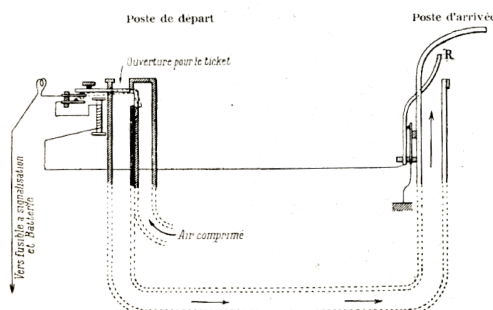
Fig. 2. — Tube pneumatique pour l'envoi des tickets.
