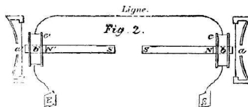
Schéma de principe (La nature de 1877)
