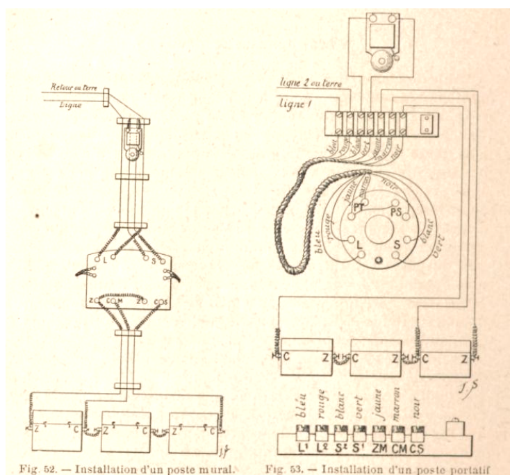
Fig. 52. — Installation d'un poste mural.
