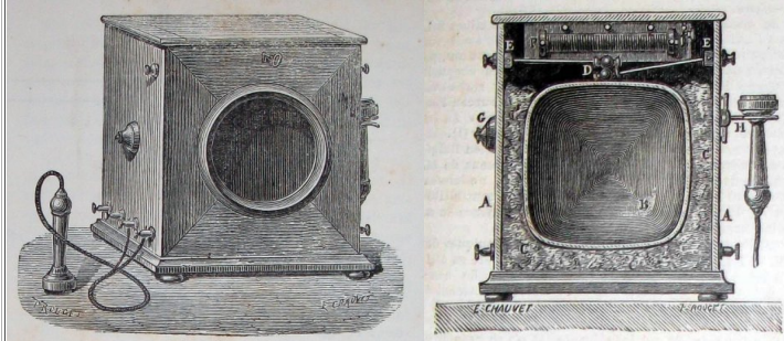
Fig. 1. — Electrophone Louis Maiche, d'après une photographie
