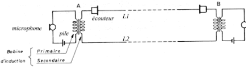
schéma de connexion entre deux postes avec piles
