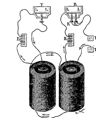
Dispositif utilisé selon le brevet Berliner
