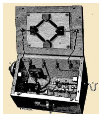
Le microphone de Crossley (à gauche) et le micro Ader
