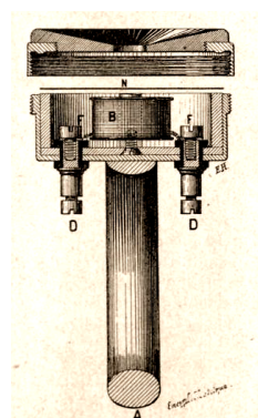
Fig. 2. — Récepteur à anneau Breguet.
